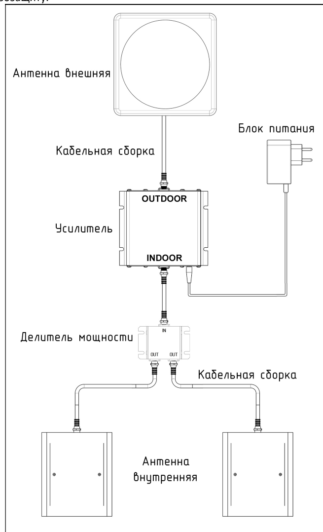
Схема 3 – Подключение комплекта
