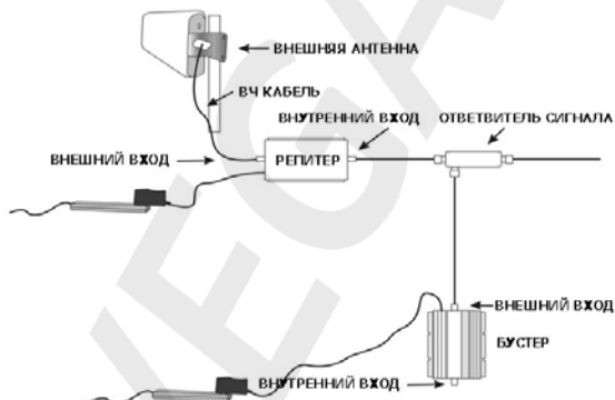
Схема подключения бустера
