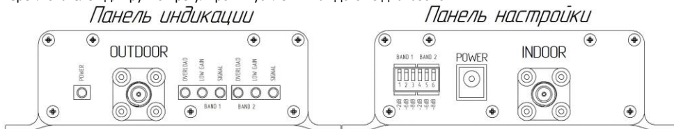
Рисунок 2 – Панели усилителя
